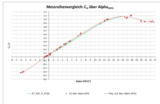
Abbildung 1: Aufgelöste Polare des ATISS mit MOWI (rot) und aus Flugleistungsvermessung (grün)
