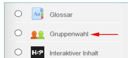
Abbildung 7: „Gruppenwahl“ auswählen
