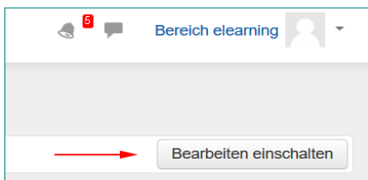
Abbildung 5: Bearbeitung einschalten
