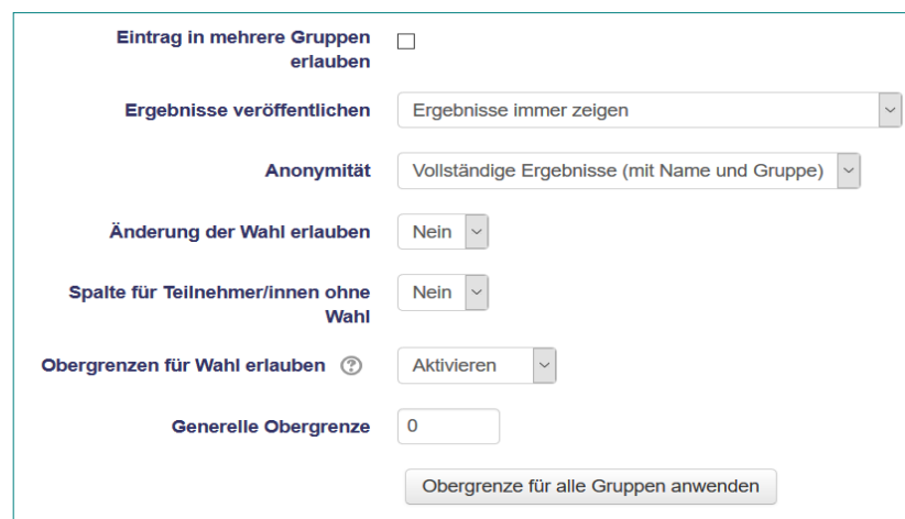
Abbildung 9: Verschiedene Einstellungen
