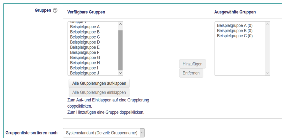
Abbildung 10: Gruppeneinstellungen
