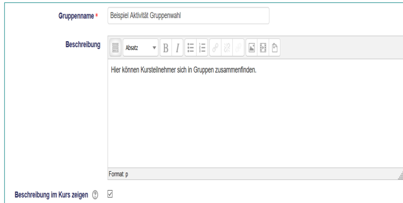
Abbildung 8: Allgemeine Einstellungen
